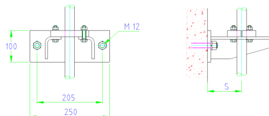
Rod guide
